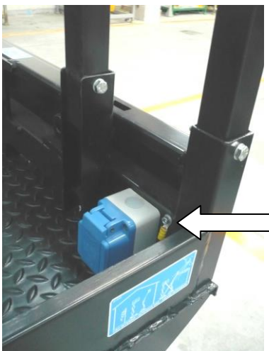
5-8: Contactdoos op hoogte
