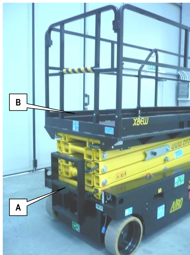
5-4: Positie voor betreden/verlaten van platform
