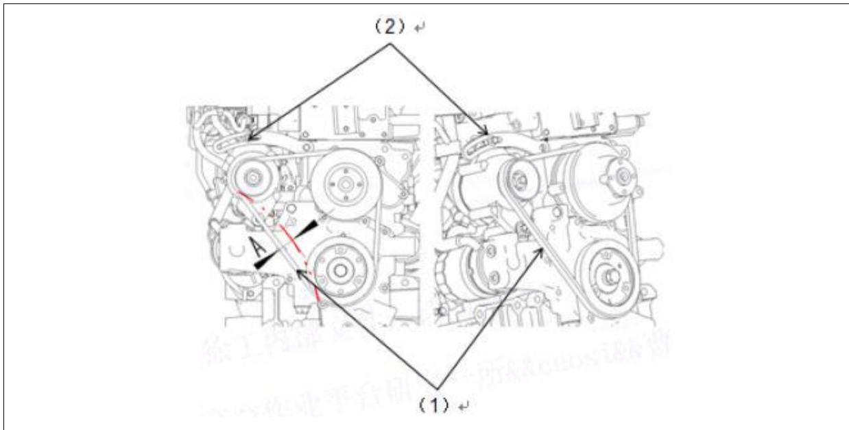
Fig.6-36 Installatie V-riem
