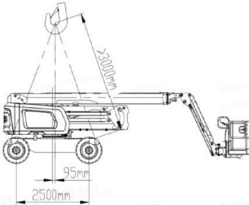
Fig. 8-5 Hijs de machine met een kraan
