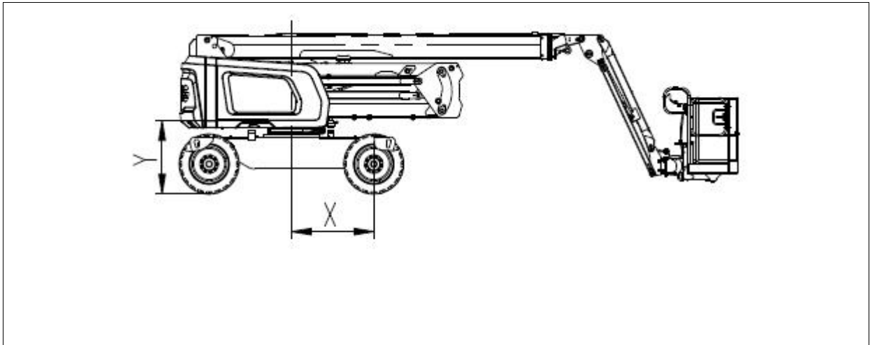
Fig. 8-1 Zwaartepunt van de machine
