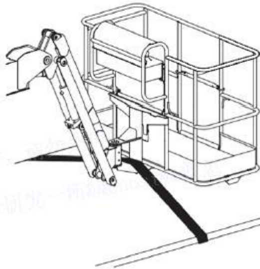
Fig. 8-3 Schematisch diagram van de bevestiging van het werkplatform tijdens transport
