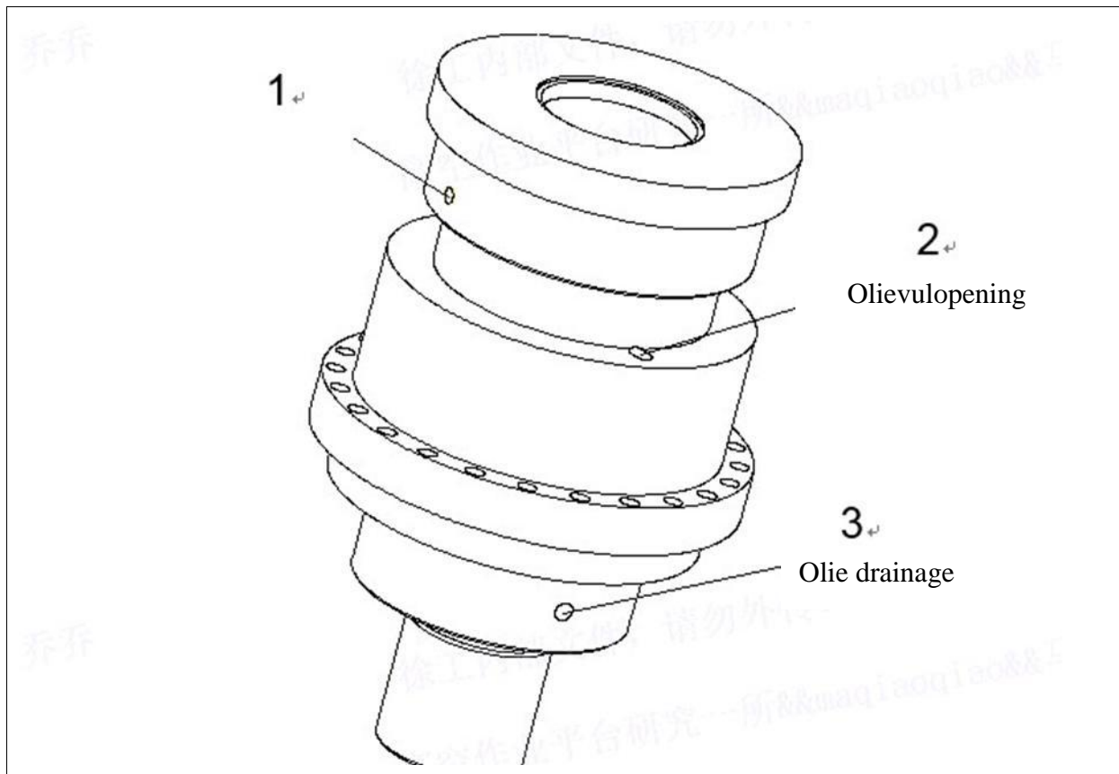
Fig.6-14 Schematisch diagram van de positie van de oliepoort van het roterende verloopstuk
