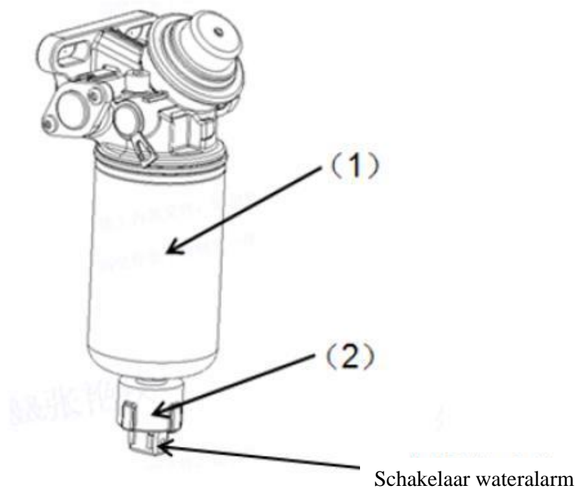
Fig. 6-26 Waterscheider
