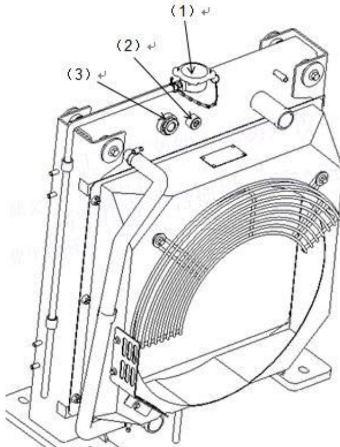
Fig. 6-33 De radiator
