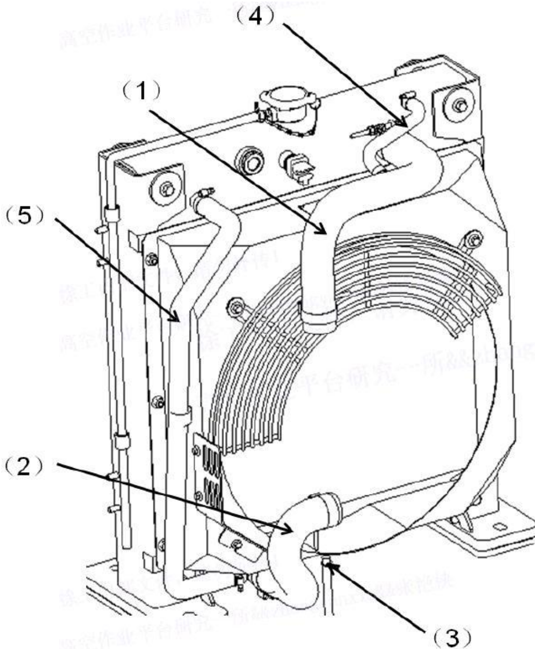
Fig.6-34 Koelsysteem leidingen (1)
