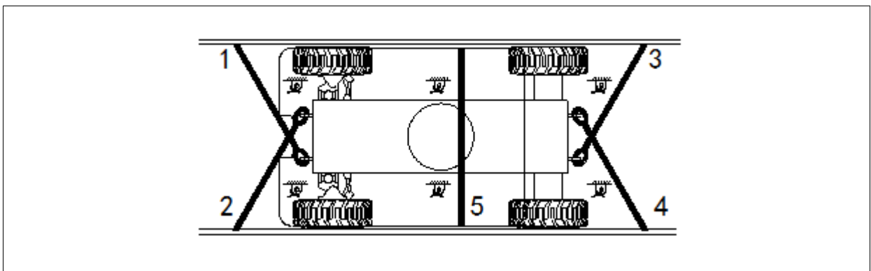
Fig. 8-2 Schematisch diagram van chassisbevestiging tijdens transport
