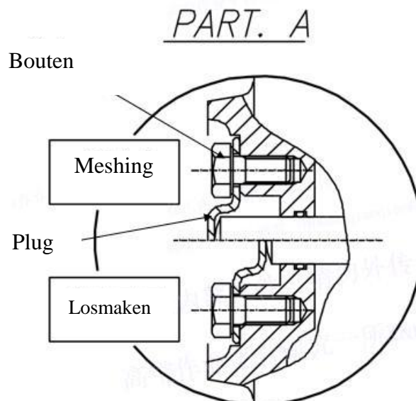
Fig.6-19 Schematisch diagram van loopreducerscheider
