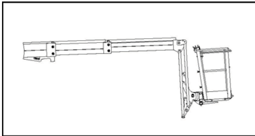
Fig. 199 Controle slijtage leisloffen uitschuifgedeelte
