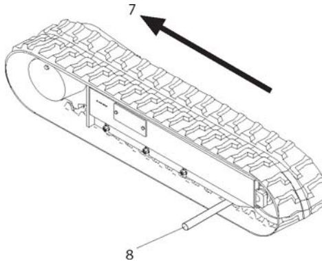
Fig. 194 Voorbeeld montage rupsband
