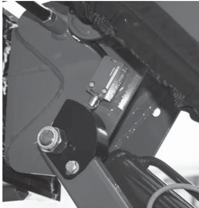
Fig. 16 Microschakelaar JIB
