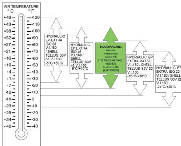
Fig. 180 Gebruikstemperaturen olie
