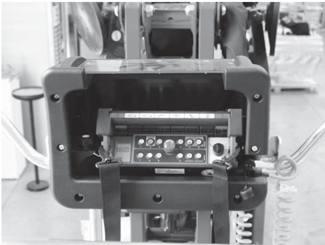
Fig. 19 Bescherming bedieningsorganen in hoogwerkerbak
