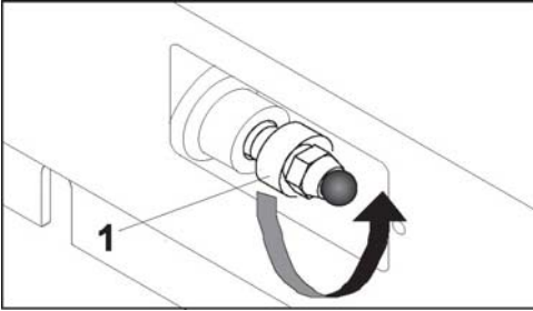
Fig. 192 Klep spanwiel
