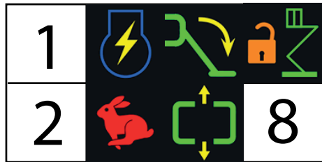
Fig. 162 Pictogram signalering bypass beveiligingen geactiveerd
