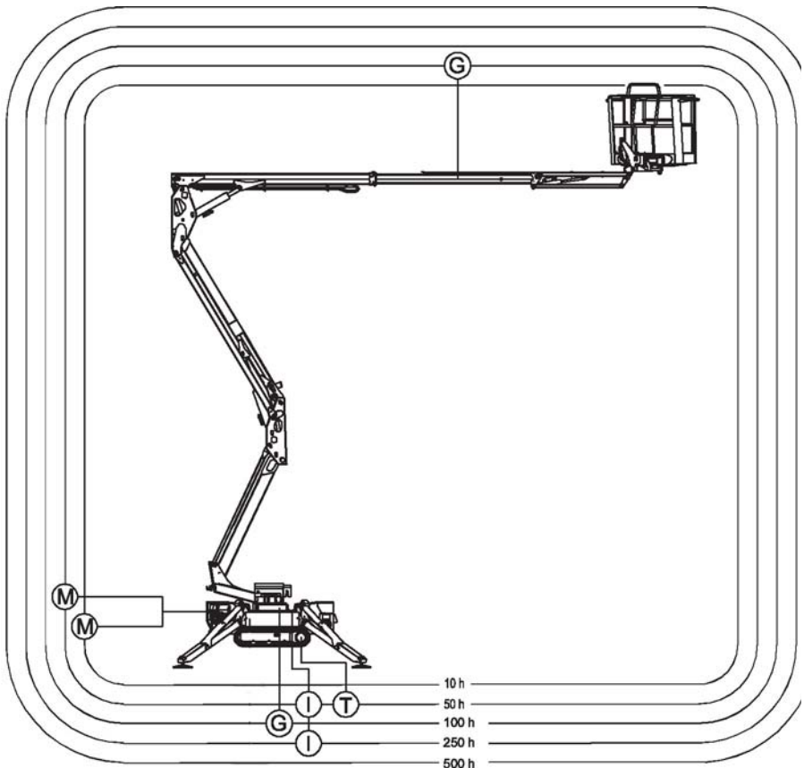
Fig. 182 Schema Smeerpunten
