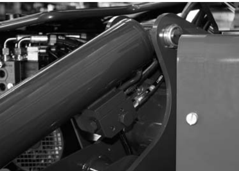
Fig. 10 Blokkeerklep stabilisatiepoten
