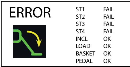
Fig. 131 Fout machine niet gestabiliseerd
