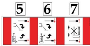
Fig. 110 Pictogrammen in de buurt van de bediening aan de grond 2
