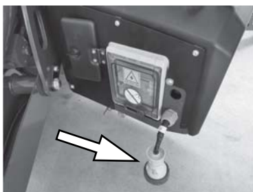
Fig. 178 Stopcontact
