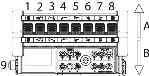
Fig. 140 Bedieningen joysticks
