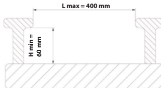
Fig. 204 Profiel oprijplank
