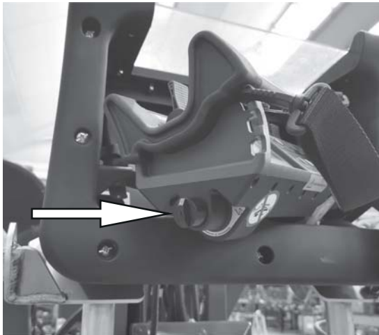
Fig. 137 Sleutel nivellering hoogwerkerbak
