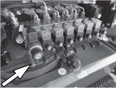
Fig. 156 Knop activering proportionele klep hoogwerkerdeel
