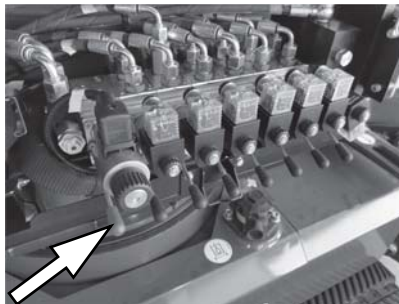
Fig. 106 Hendel activering proportionele klep bovenbouw
