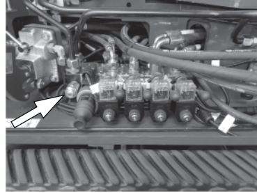
Fig. 9 Overdrukklep onderstel
