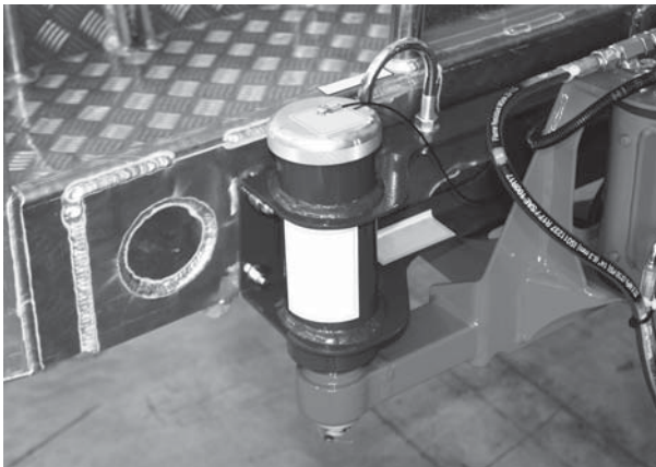
Fig. 202 Pen blokkeerdeksel
