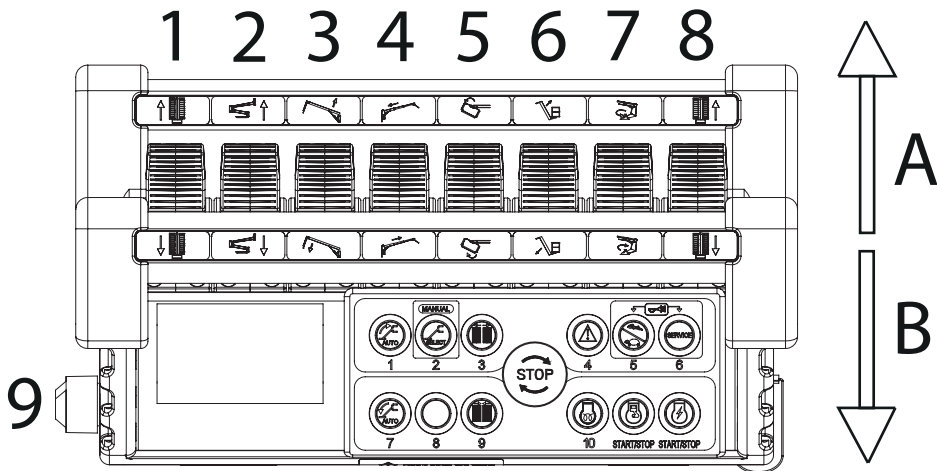
Fig. 65 Bedieningen joysticks
