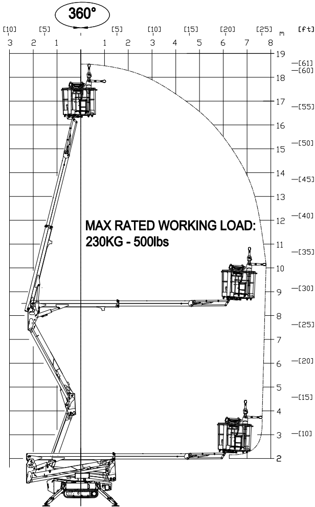
Fig. 111 Werkgebied
