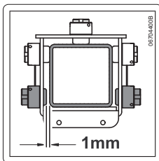
Fig. 200 Sticker laat 1mm alleen op de onderste zijdelingse leisloffen
