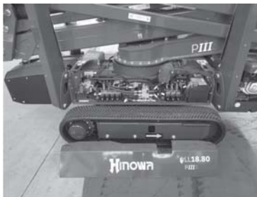
Fig. 147 Ruimte elektrische/hydraulische componenten
