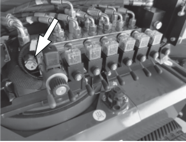
Fig. 8 Overdrukklep bovenbouw
