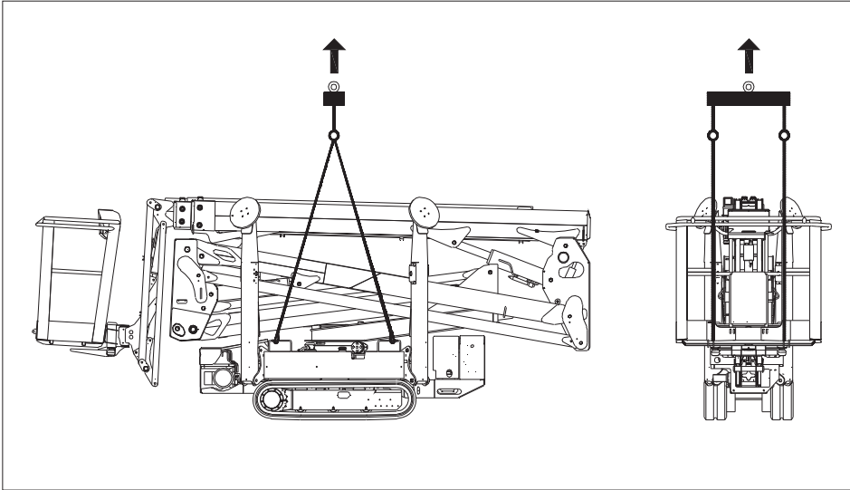
Fig. 207 Hijsschema met kabels of kettingen
