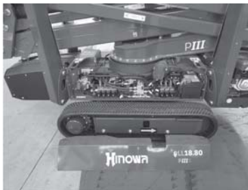
Fig. 163 Ruimte elektrische/hydraulische componenten
