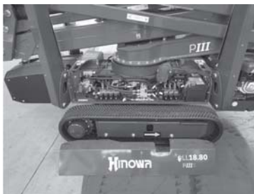
Fig. 158 Ruimte elektrische/hydraulische componenten
