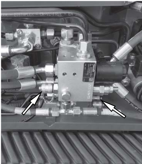
Fig. 198 Drukaansluitingen op de machine
