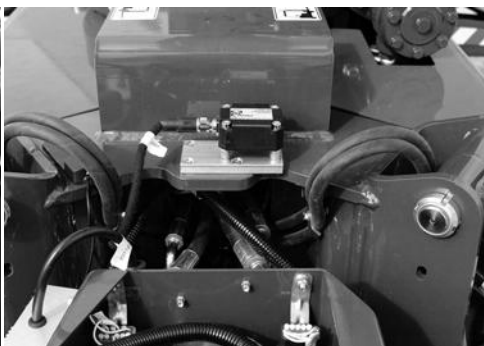
Fig. 23 Inwendige elektronische luchtbel
