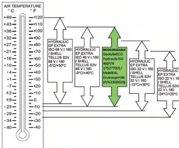
Fig. 152 Gebruikstemperaturen olie
