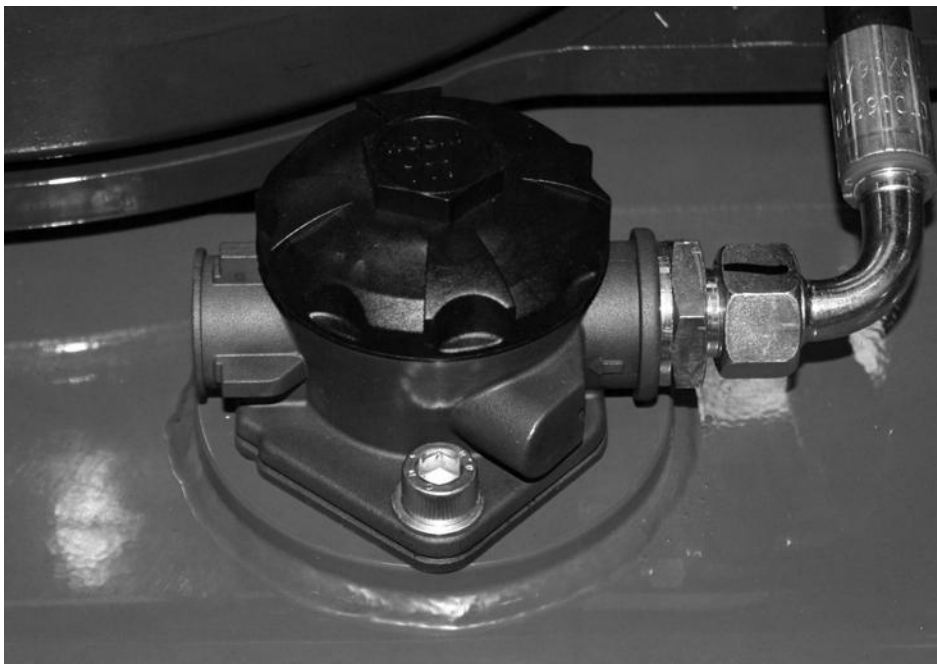
Fig. 169 Positie filter hydraulische olie
