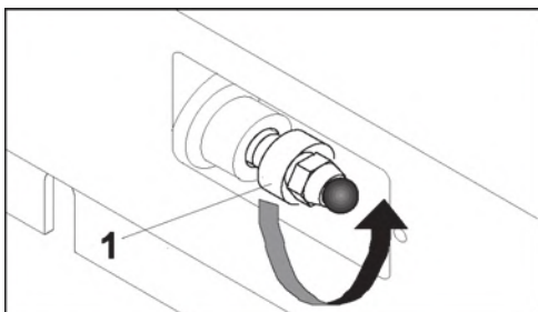
Fig. 163 Klep spanwiel
