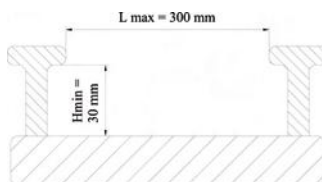
Fig. 174 Profiel oprijplank
