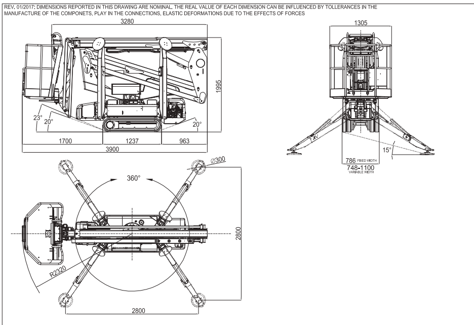
Fig. 5 Standaardversie met tweepersoonsbak
