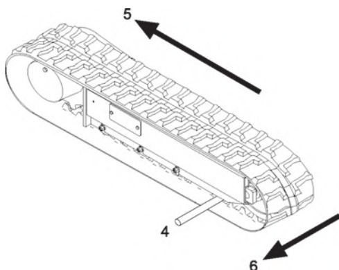
Fig. 165 Voorbeeld demontage rupsband
