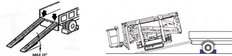
Fig. 173 Met oprijplanken laden
