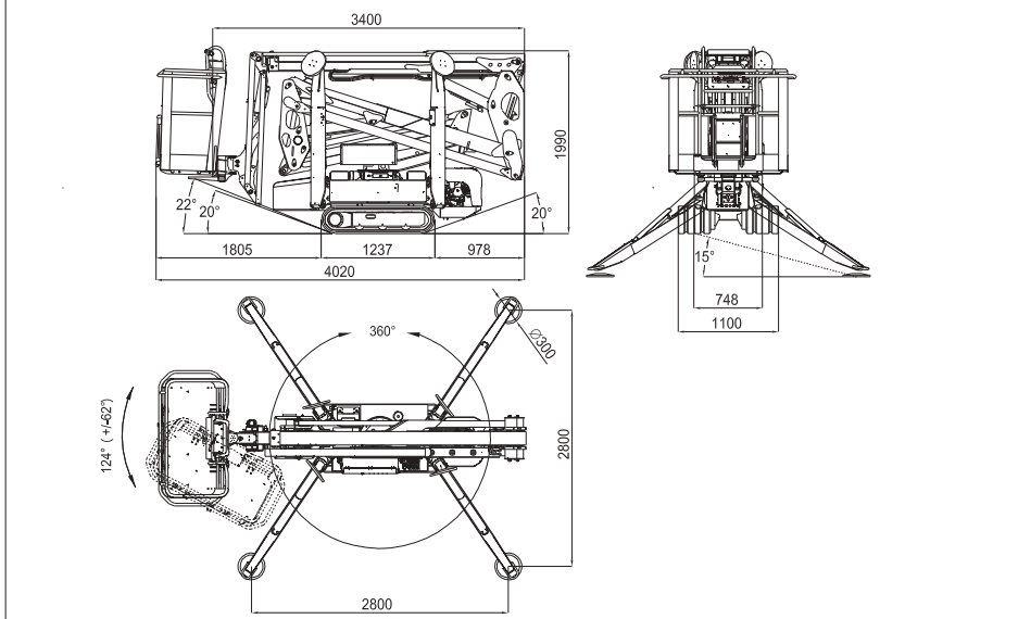
Fig. 4 Standaardversie met tweepersoonsbak
