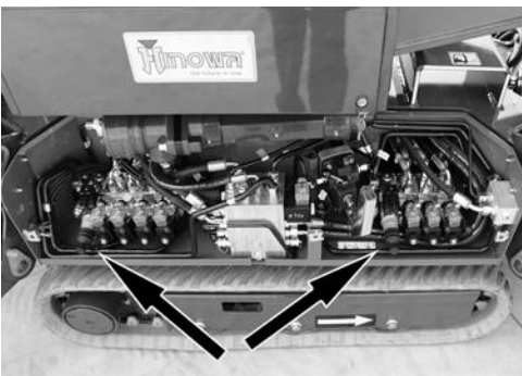
Fig. 143 Knoppen activering proportionele klep wagendeel
