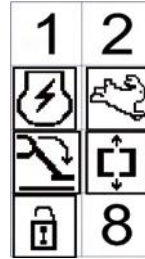
Fig. 138 Pictogram signalering bypass beveiligingen geactiveerd
