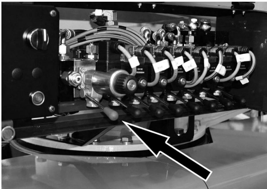
Fig. 76 Knop activering proportionele klep hoogwerkerdeel
