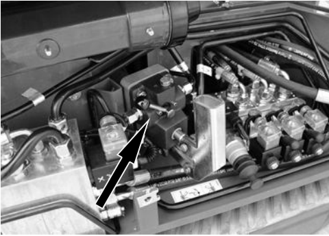
Fig. 141 Handbediende tuimelschakelaar handpomp
