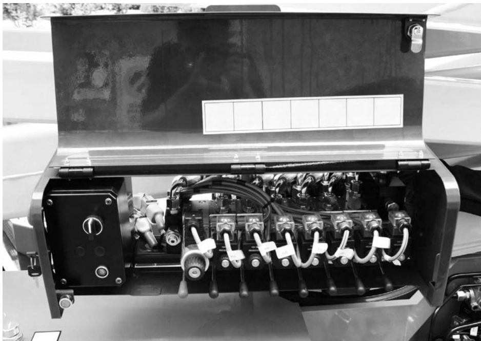
Fig. 74 Bedieningen op verdeler hoogwerkerdeel
