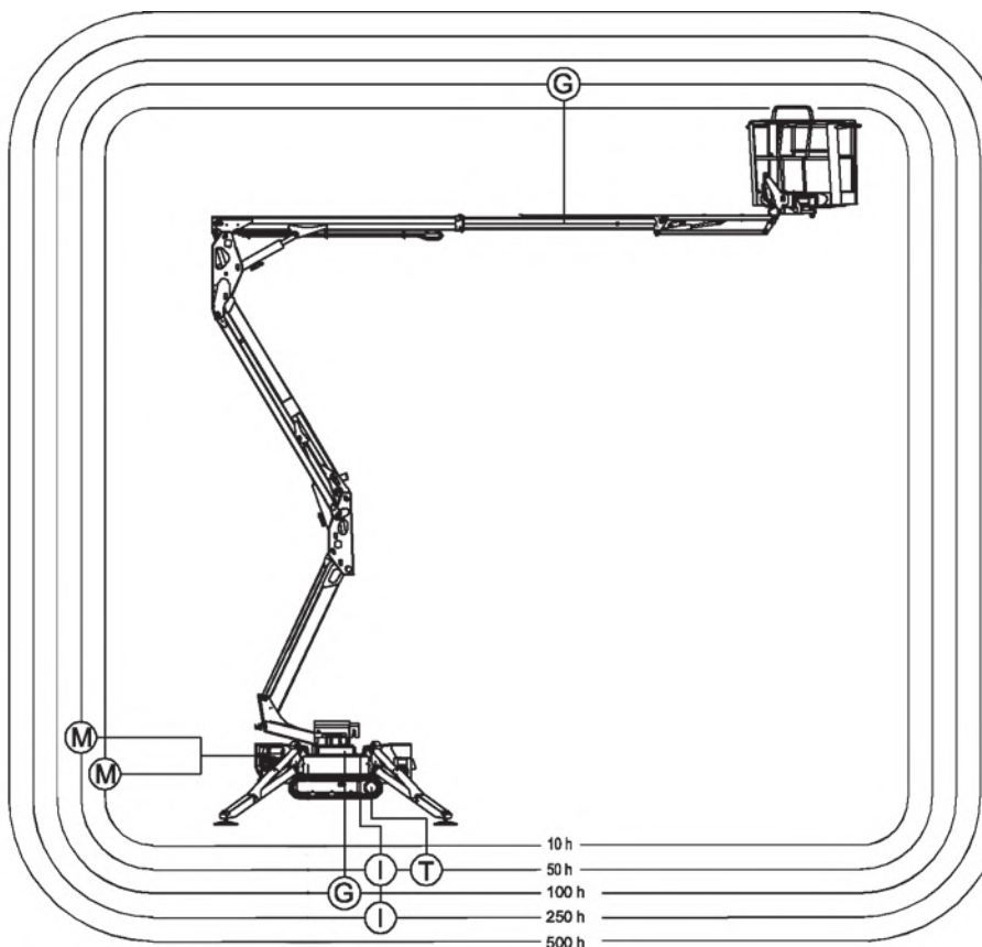
Fig. 154 Schema Smeerpunten
