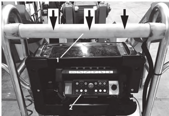
Fig. 61 1-Sensor SkyGuard™ 2-SkyGuard™ By-pass (knop nummer 8)
