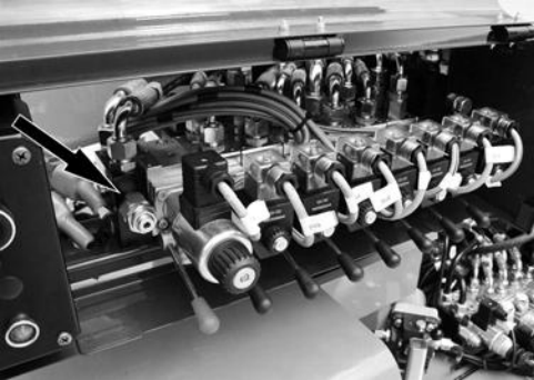
Fig. 10 Overdrukklep hoogwerkerdeel
