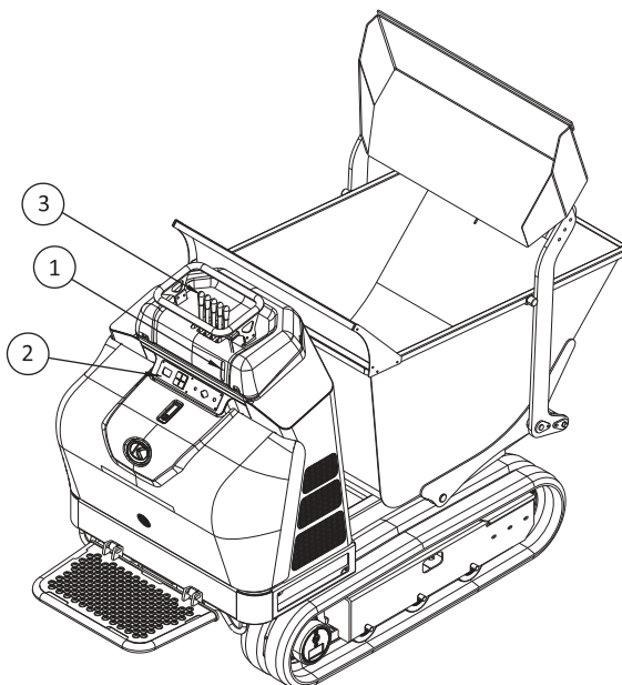
Fig. 10 Positie van de bedieningsorganen
