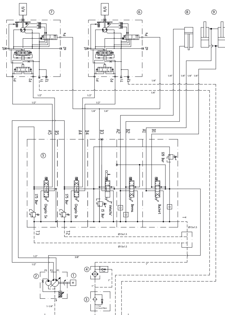
Fig. 15 Hydraulisch schema
