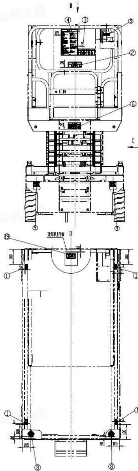
Fig. 5-8.XG1012AC labels 2/2
