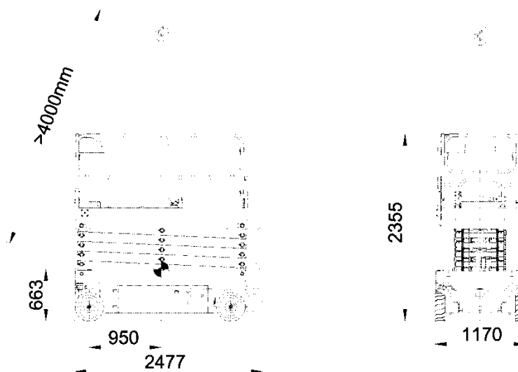
Fig. 6-3 Schematisch diagram van hijspunt
